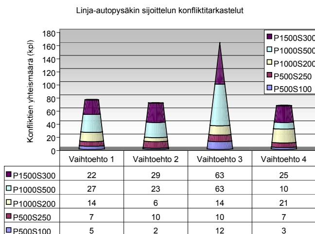
Kuva 56. Linja-autopysäkin sijainnin vaikutus konfliktimääriin.
