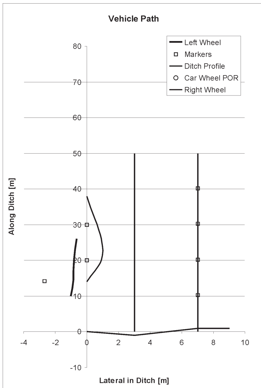
Test 9. Ford Fiesta, 81 km/h 9,0 °
