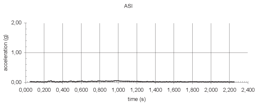
Test 4. Mercedes Benz 200 D (123), 81 km/h, 3,6 °
