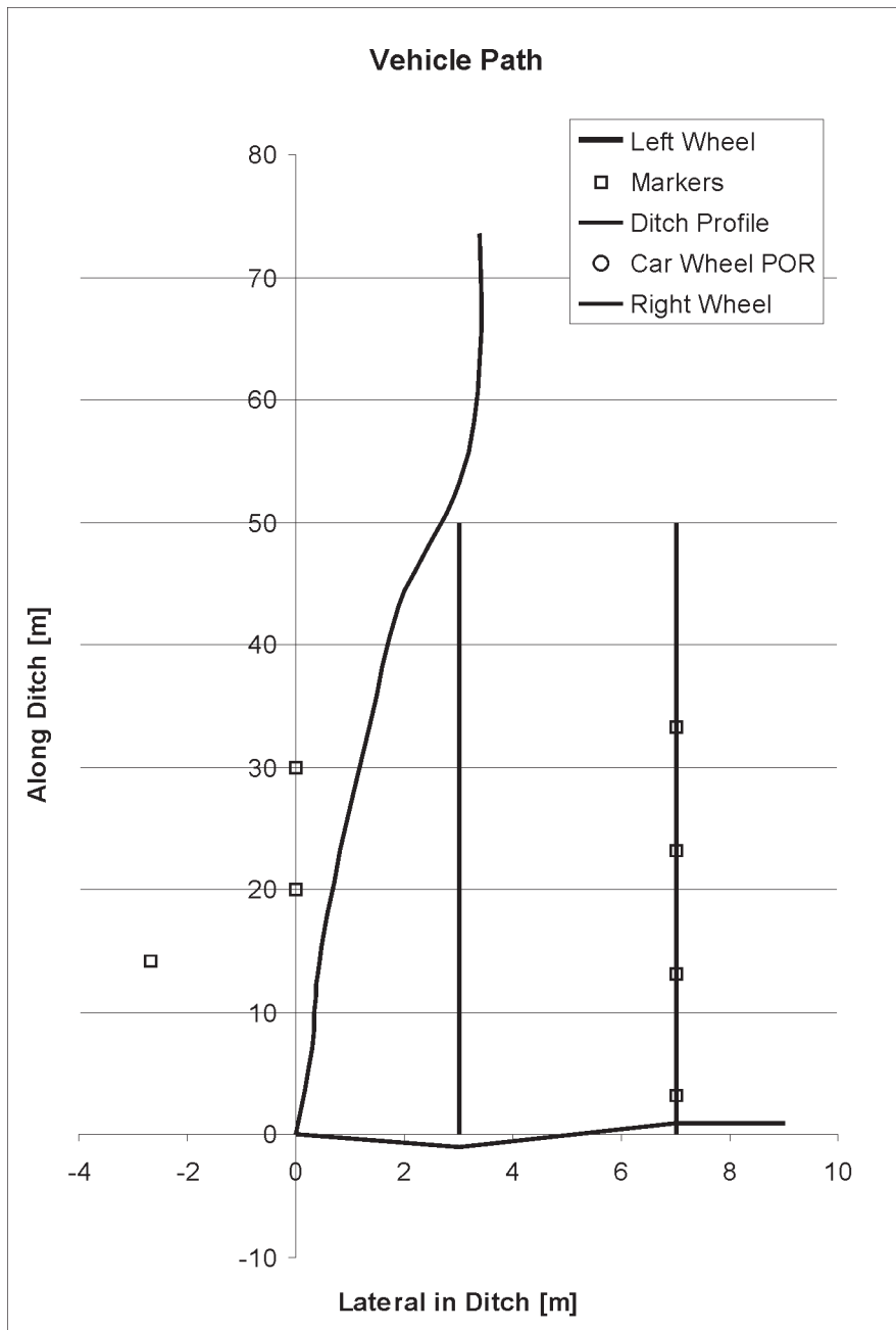
Test 2. Peugeot 205, 78 km/h, 3°
