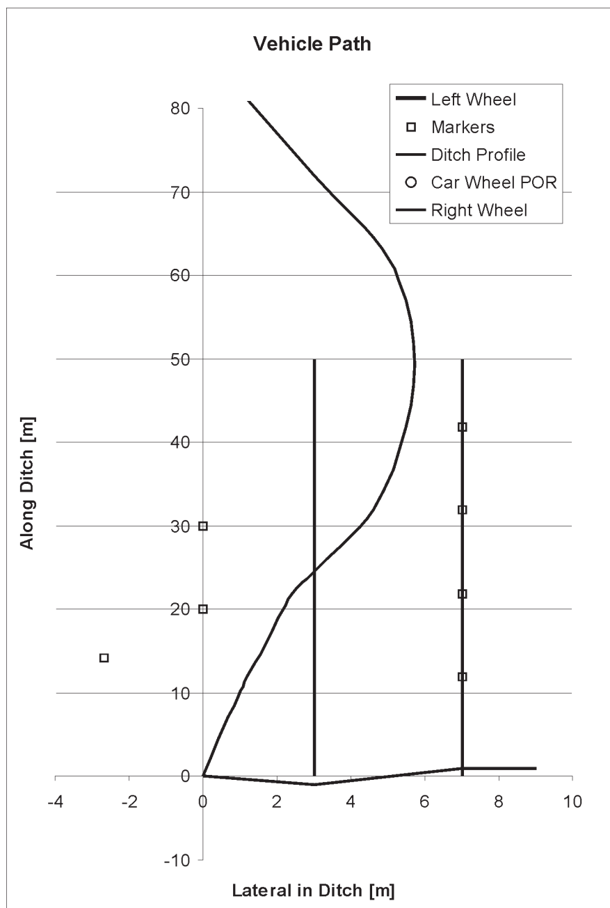
Test 3. Peugeot 205, 102 km/h, 5,7 °
