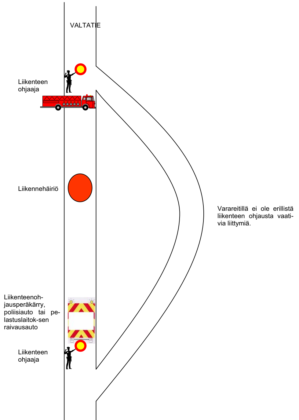
Kuva 3 Liikenteen ohjauksen järjestäminen häiriötilanteessa, kun varareitillä ei ole erillisiä ohjausta vaativia liittymiä.
