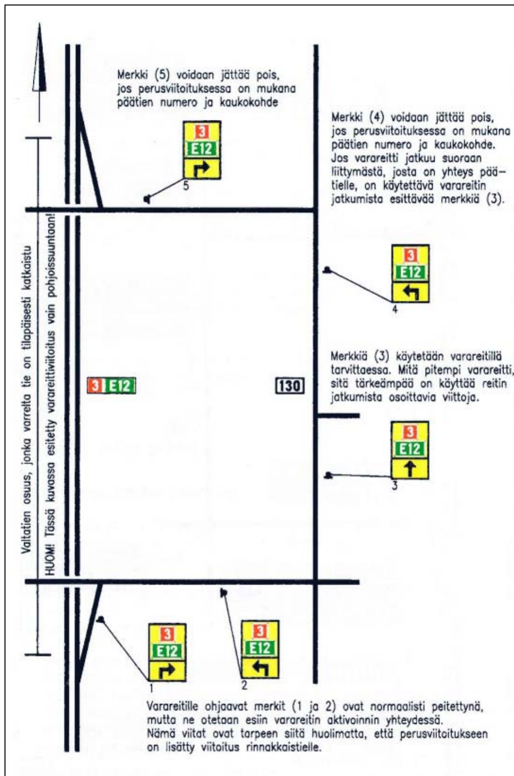
Kuva 6. Varareitin ohjausjärjestelyt moottoritien rinnakkaistiellä (Österman (1999)).
