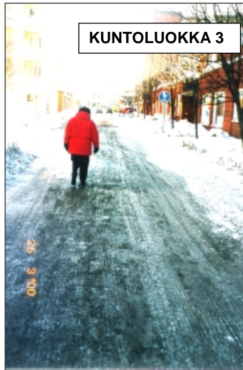
Kuva 46. Väylän pinta on karhennettu ennen hiekoittamista. Vaikka väylän pinta on jäinen, tutkimusryhmäläisten antamien arvosanojen KA = 3,29 oli yli tyydyttävän tason. Kuntoluokka = 3. Kuntoluokkaa alentavat tekijät: liukkaus 18/24, epätasaisuus 9/24.
