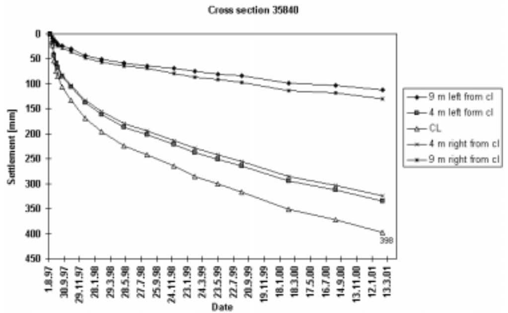
Kuva 5a. Haarajoen koepenger. Havaittu painumisnopeus. Maanvarainen penger.
