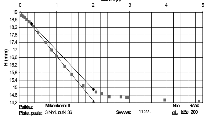
AIKA-PAINUMA- KUVAAJA, TAYLOR SQRT t (h)
