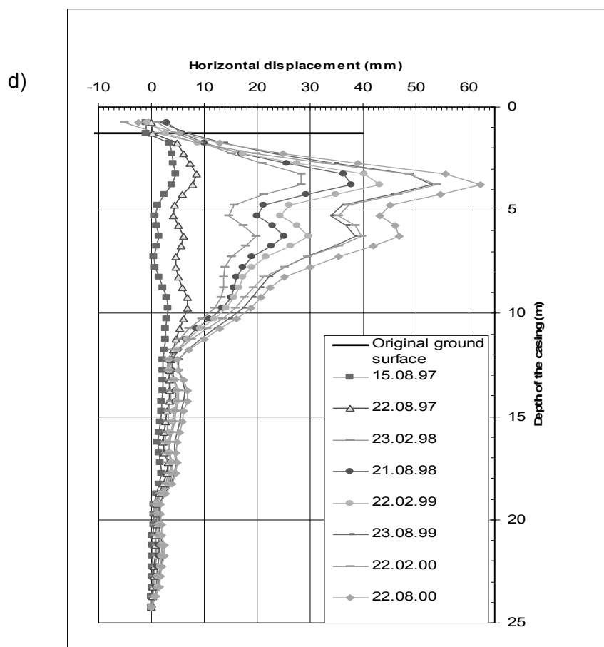
Kuva 7. Haarajoen koepenger. c) Maanpinnan siirtymä ja maksimisiirtymä. d) Havaittu sivusiirtymä. Inklinometri I2. Maanvarainen pengger.
