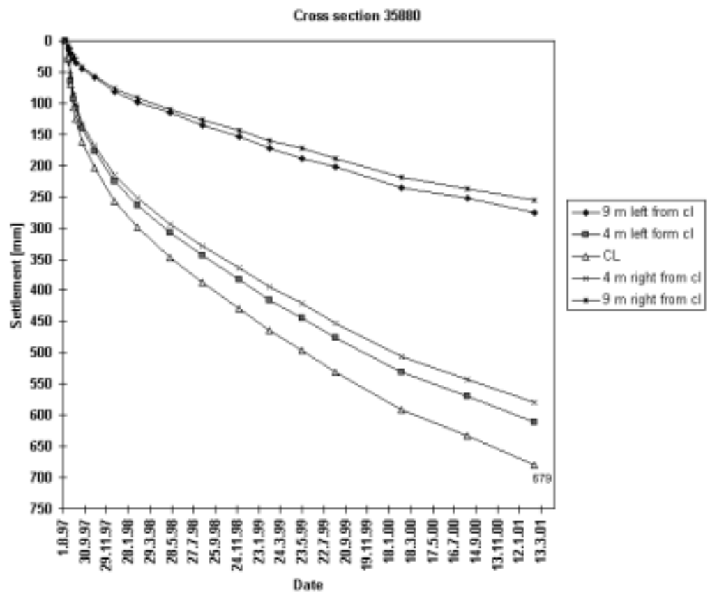
Kuva 5b. Haarajoen koepenger. Havaittu painumisnopeus. Pystyjitettu penger.
