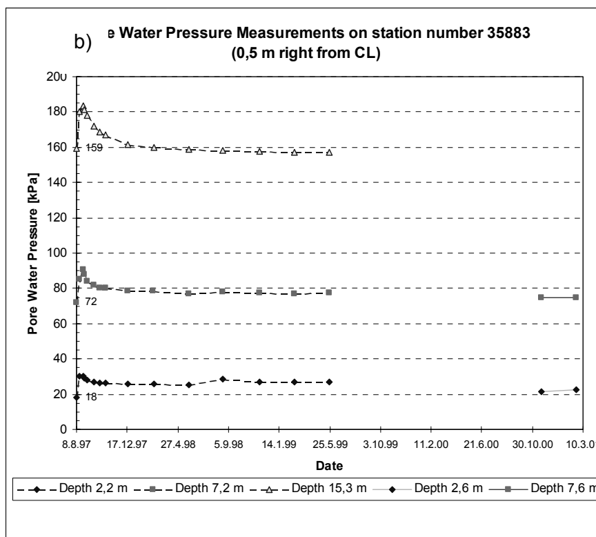
Kuva 6. Haarajoen koepenger. Havaittu huokosvedenpaine. a) Maanvarainen pengerr. b) Pystyöjitettu pengerr.
