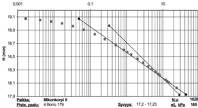
AIKA-PAINUMA- KUVAAJA, CASAGRANDE LOG t (h)
