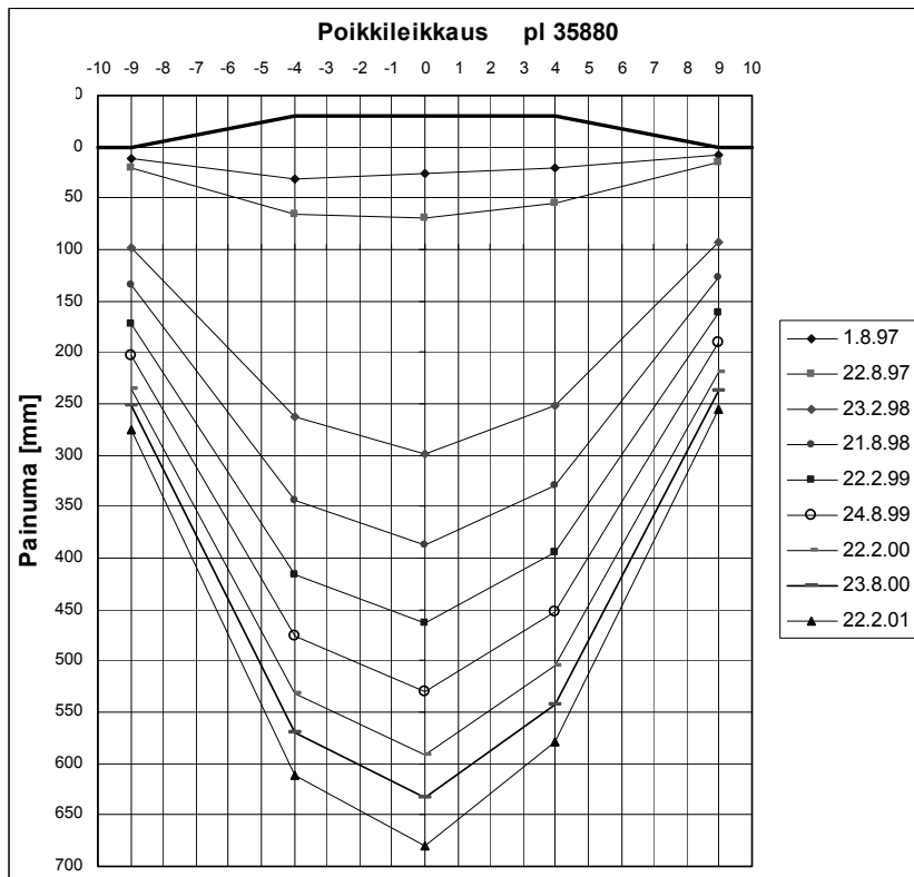
Kuva 4b. Haarajoen koepenger. Painumahavainnot. Pystyjitettu pohja.
