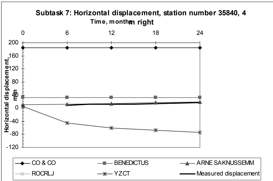
Kuva 11. Haarajoen koepenger. Laskentatulosten vertailu. Kilpailuosa 3. Sivusiirtymä. Maanvarainen pengerr.
