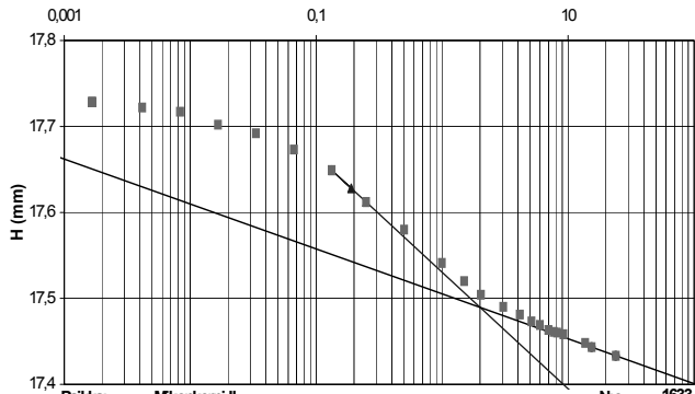
AIKA-PAINUMA-KUVAAJA, CASAGRANDE LOG t (h)
