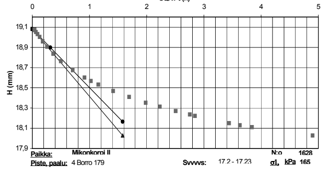
AIKA-PAINUMA- KUVAAJA, TAYLOR SQRT t (h)
