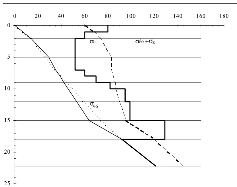
Kuva 3. Haarajoen koepenger. Jännitysjakaumat savikerroksissa. Vallitseva jännitys on merkitty katkoviivalla, \sigma'_{vo} on vallitseva tehokas jännitys, \sigma_z on lisäjännitys ja \sigma'_c on portaittaisesta ödometrikokeesta määritetty esikonsolidaatiojännitys. [Saarelainen 1997]
