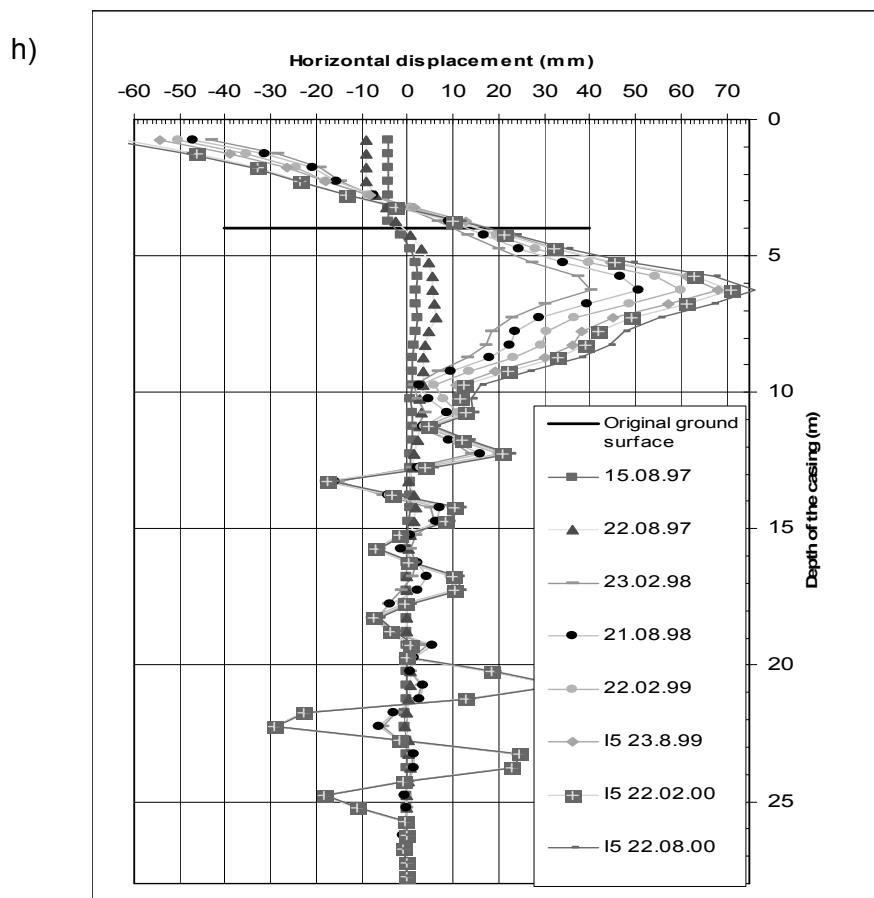
Kuva 7. Haarajoen koepenger. g) Maanpinnan siirtymä ja maksimisiirtymä. h) Havaittu sivusiirtymä. Inklinoimetrit I1 ja I5. Maanvarainen pengerr.
