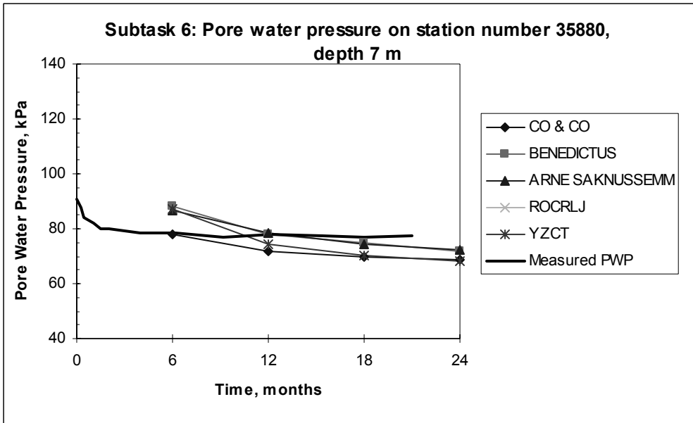
Kuva 14. Haarajoen koepenger. Laskentatulosten vertailu. Pystyjitettu penger. Huokosvedenpaine 7 m:n syvyydessä. Kilpailuosaa 3.
