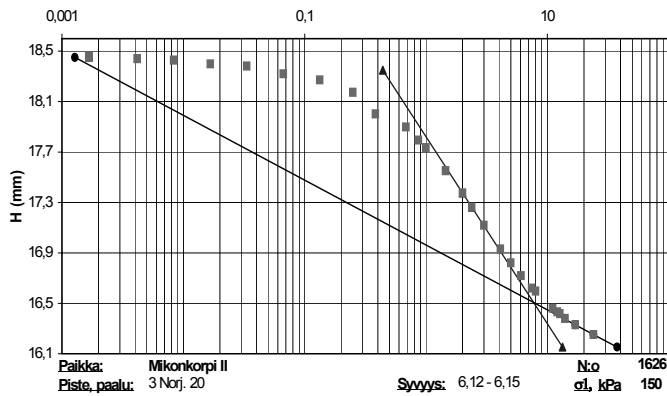
AIKA-PAINUMA- KUVAAJA, CASAGRANDE LOG t (h)
