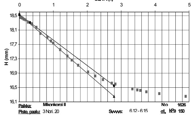
AIKA-PAINUMA- KUVAAJA, TAYLOR SQRT t (h)
