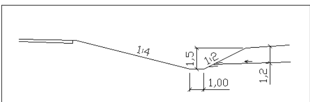
Kuva 7: Putkitettu oja, sisäluiskan leveys vaihtelee tiettyyn mukaan ( \geq 2 m)
