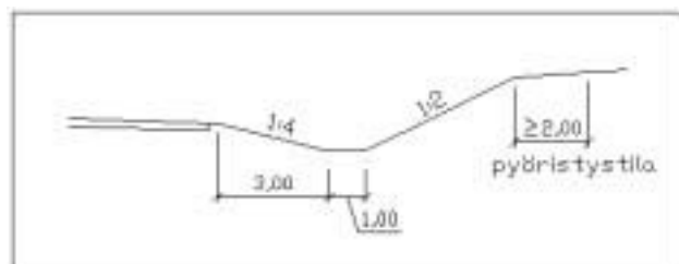
Kuva 3: Maaleikkaus.
