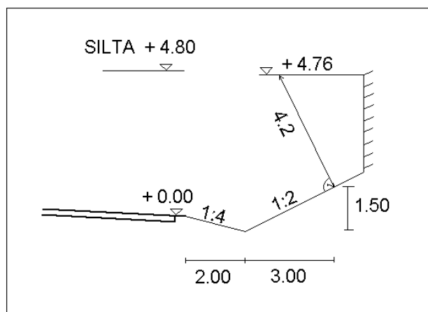
Kuva 14: Vapaan tilan korkeus turvallisuusalueella. Siltojen, portaalien ja muiden tien ylittävien rakenteiden kohdalla vaadittava vapaan tilan korkeus (4,8 m) määritellään turvallisuusalueella siten, että ulkoluiskaa (1:2) vastaan kohtisuoraan mitattuna tulee olla 4,2 metrin vapaa korkeus. Vaatimus on kuitenkin voimassa vain 1,5 m korkeuteen asti ojan pohjasta. Portaalit ja siltipilarit voidaan myös sijoittaa turvallisuusalueelle, kun ne suojataan kaiteella. Tällöin vapaan tilan korkeusvaatimukset ovat voimassa vain kaiteen toimintaleveyden määrittämällä alueella. Pilarien sijainnissa on otettava huomioon tien tulevat leventämistarpeet.
