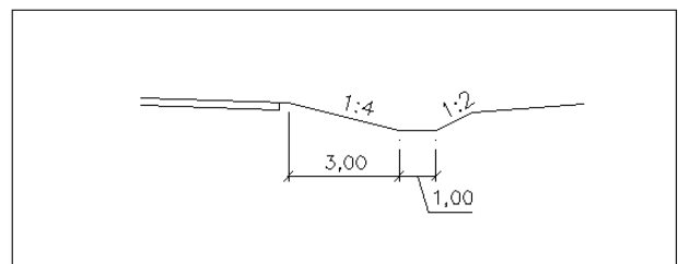
Kuva 2: Tien tasaus lähellä maanpintaa.
