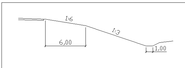
Kuva 6: Levennetty pengerr (1:6/1:3)
