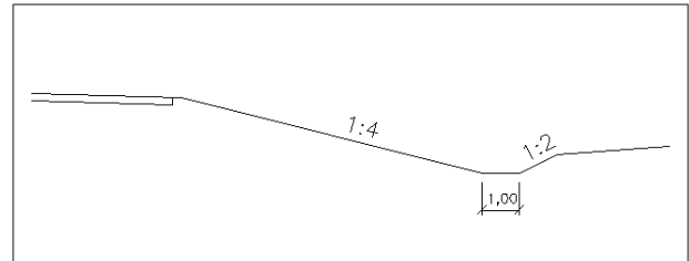
Kuva 1: Kaiteeton penger, vaihtoehtoisesti voidaan tehdä jyrkkä oja 2 – 6 metrin etäisyydelle luiskan alareunasta (etäisyys riippuu tien nopeudesta ja liikennemäärästä, kohdan 3 mukaisesti).
