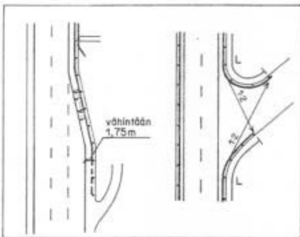
Kuva 21: Kaiteen aloittaminen pysäkin kohdalla ja kaiteen päiden kääntäminen vähäliikenteiselle sivutielle.
