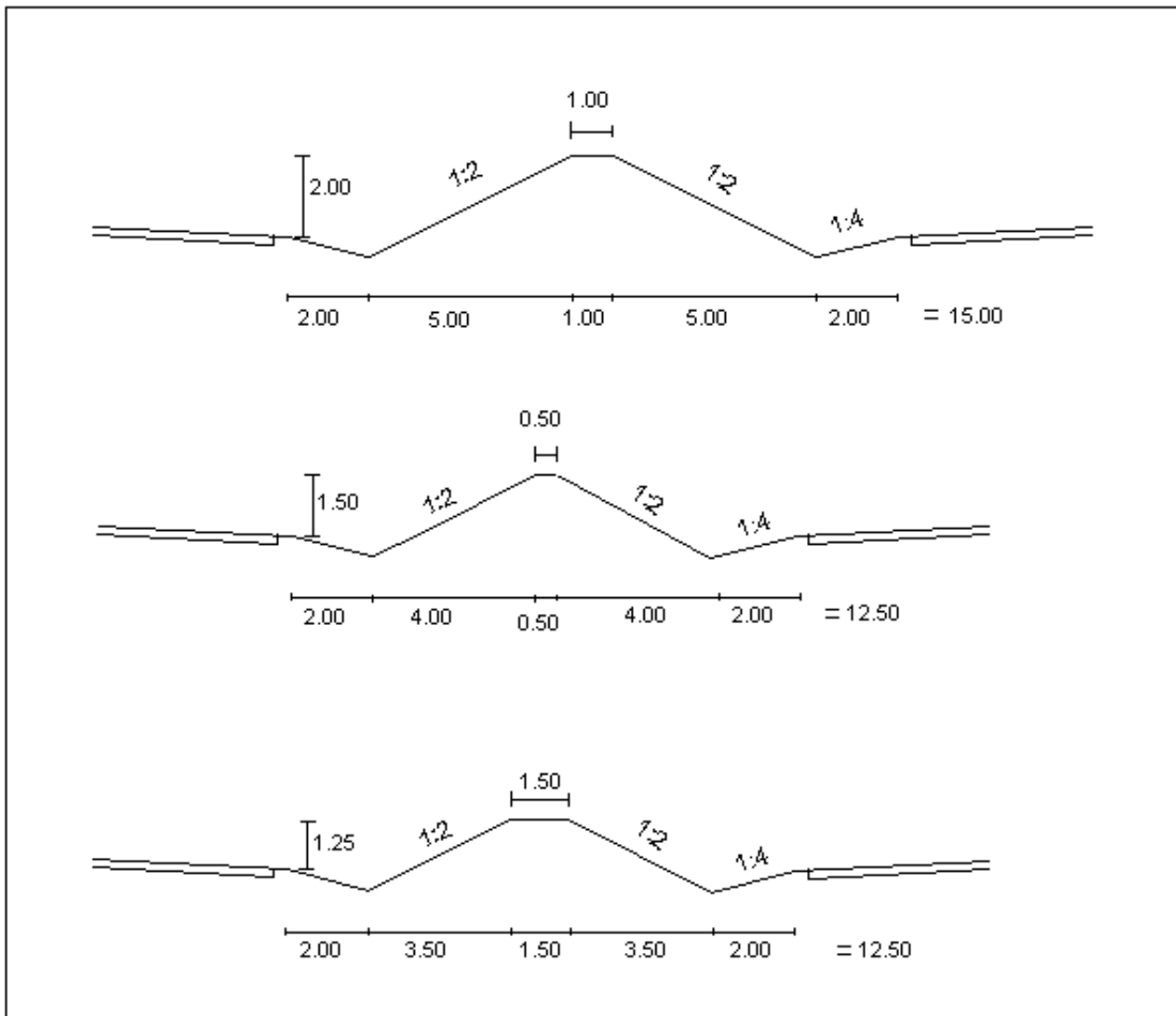
Kuva 16: Valli keskialueella.
