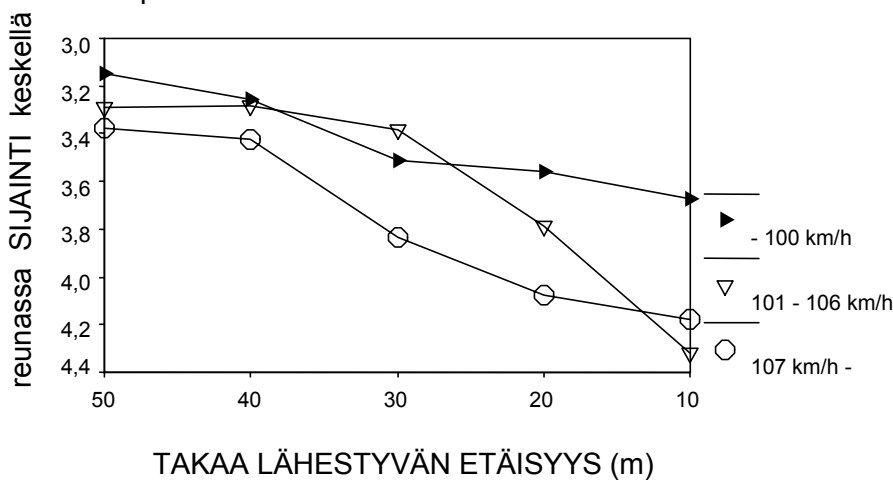
Kuva 8. Alkutilanteessa (n. 100 m:n etäisyydellä) keskellä kaistaa ajaneiden keskimääräinen sijainti nopeusluokittain ohittavan ajoneuvon etäisyyden funktiona.
