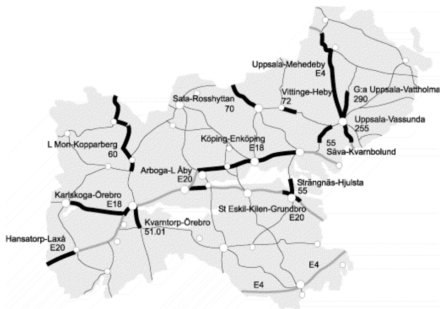
Kuva 3. Ruotsin koetie E 18 Köping – Enköping (keskellä kuvaa).
