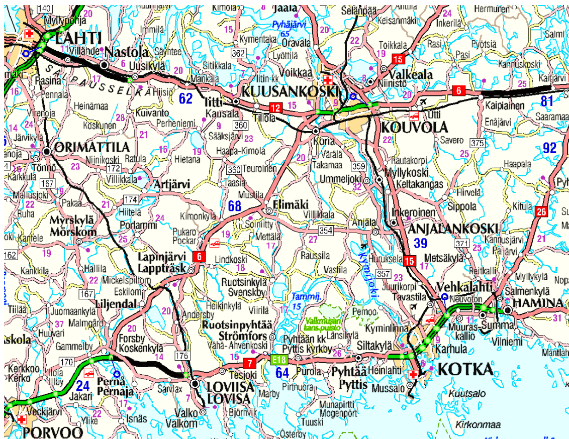
Kuva 2. Suomen koetiet (tummalla merkityt): vt 12 Lahti - Uusikylä (1995); vt 7 Koskenkylä - Loviisa (1998); vt 6 Kaipiainen - Kaitjärvi (1999).
