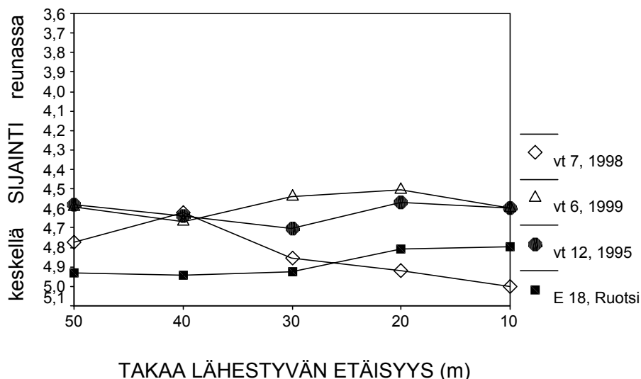
Kuva 9. Raskaiden ajoneuvojen keskimääräinen sijainti eri tutkimusteillä ohittavan ajoneuvon etäisyyden funktiona.
