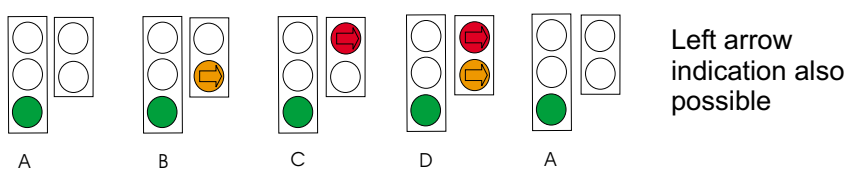
Figure 2.2: Allowed lense arrangements in Finland (Kehittämiskeskus 1996)
