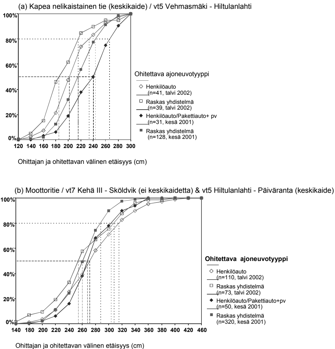
Kuva 9. Ohittavan ja ohitettavan ajoneuvon välinen etäisyys (a) kapealla nelikaistaisella tiellä ja (b) moottoritieellä kesä- ja talviolosuhteissa.
