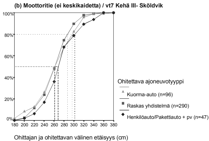
Kuva 5. Ohittavan ja ohitettavan ajoneuvon välinen etäisyys kapealla nelikaistaisella tiellä (a) ja moottoritieellä valtatiellä 7 (b) kesäolosuhteissa. Kaikissa tilanteissa ohittajana oli henkilöauto.
