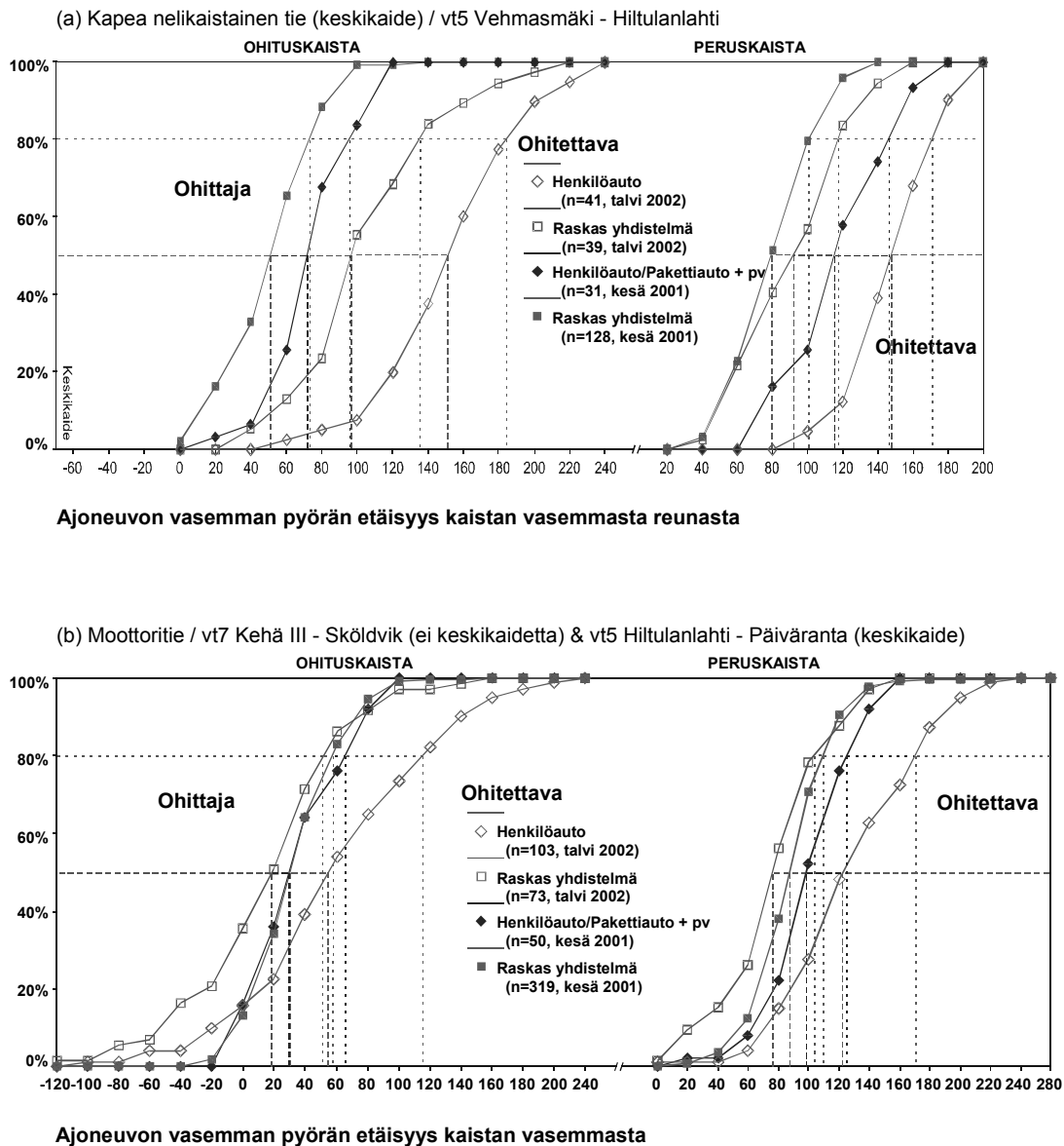
Kuva 8. Ajoneuvojen sijaintijakaumat ohitustilanteissa kapealla (a) nelikaistaisella tiellä ja (b) moottoritiellä kesä- ja talviolosuhteissa.
