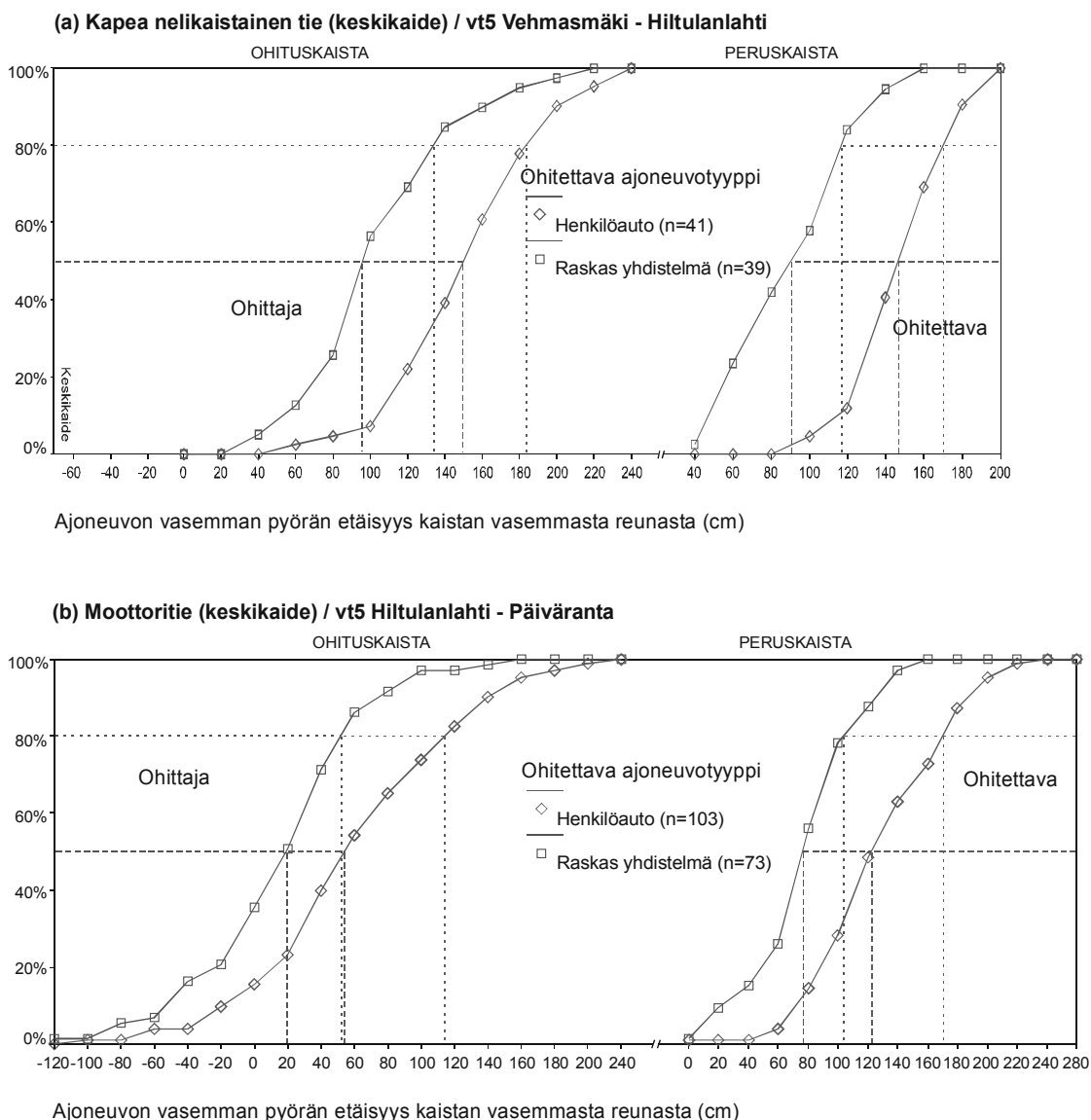
Kuva 6. Ajoneuvojen sijaintijakaumat ohitustilanteissa kapealla (a) nelikaistaisella tiellä ja (b) moottoritiellä valtatiellä 4 talviolosuhteissa. Kaikissa tilanteissa ohittajana on henkilöauto.
