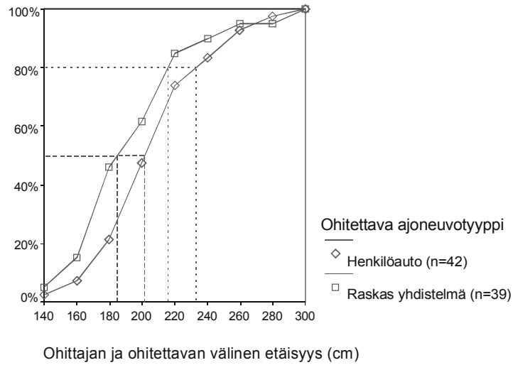
(a) Kapea nelikaistainen tie (keskikaide) / vt5 Vehmassäki - Hiltulanlahti
