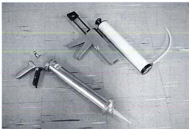
Kuva 1. Saumauspistooleja.
