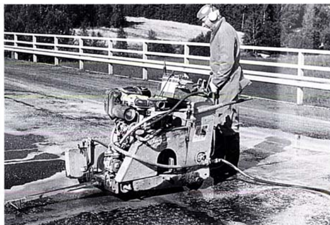
Kuva 3. Päällysteen saumausuran leikkausta.
