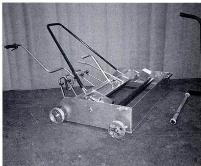
Kuva 6. Kerminasennusvaunu ja rullankelauslaite
