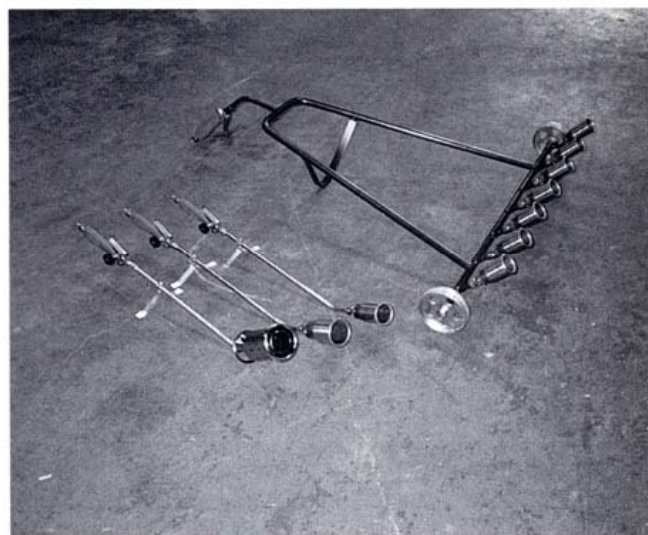
Kuva 7. Käsipolttimia ja rivipoltin
