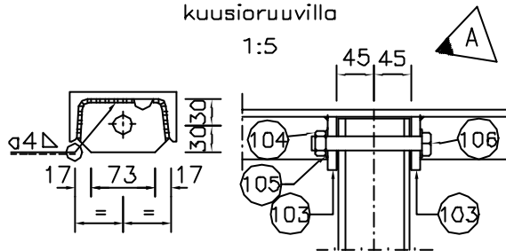
Yläjohteen kiinnitys pylvääseen kuusioruuvilla
