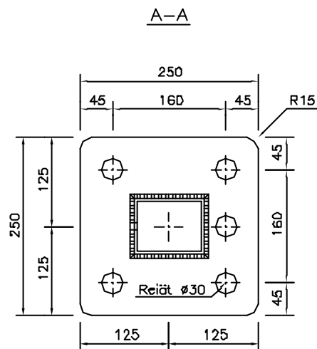
Kiinnityspultti osa 3
