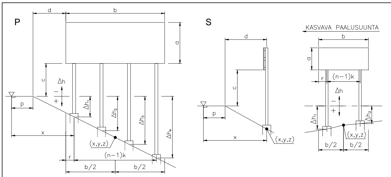
Kuva 1.1 Laskennassa käytettävät mittasuureet. Vasemmalla tapaus, jossa taulu on sijoitettu kohtisuoraan tietä vastaan (pätiemerkki = P). Oikealla tapaus, jossa taulu on sijoitettu tien suuntaisesti (sivutiemerkki = S).
