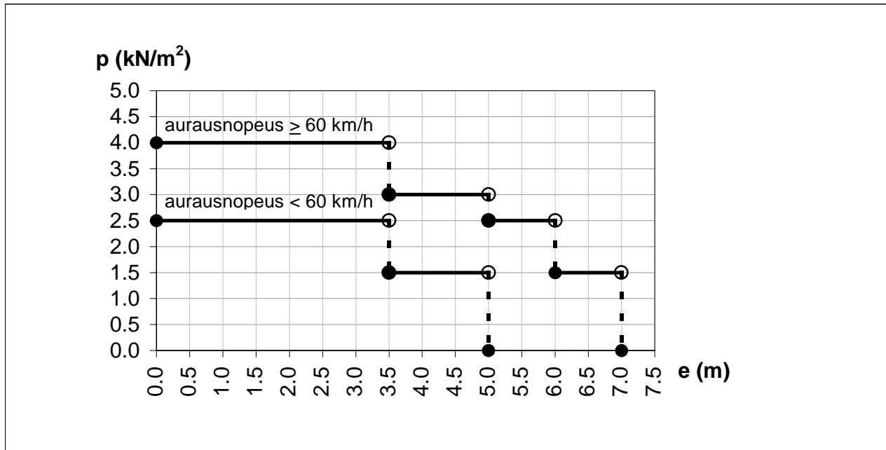
Kuva 2 Aurauskuorman intensiteetin suuruus etäisyyden funktiona vakio-
