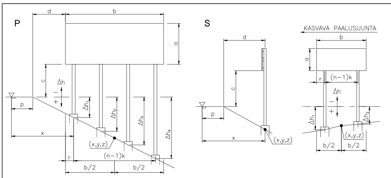
Kuva 1 Laskennassa käytettävät mittasuureet. Vasemmalla tapaus, jossa taulu on sijoitettu kohtisuoraan tietä vastaan (päätimerkki = P). Oikealla tapaus, jossa taulu on sijoitettu tien suuntaisesti (sivutiimerkki = S).
