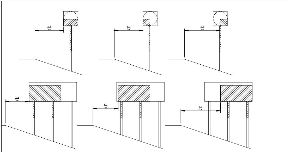
Kuva 3 Esimerkki aurasuorman laskennassa tutkittavista kuormitustilanteista.
