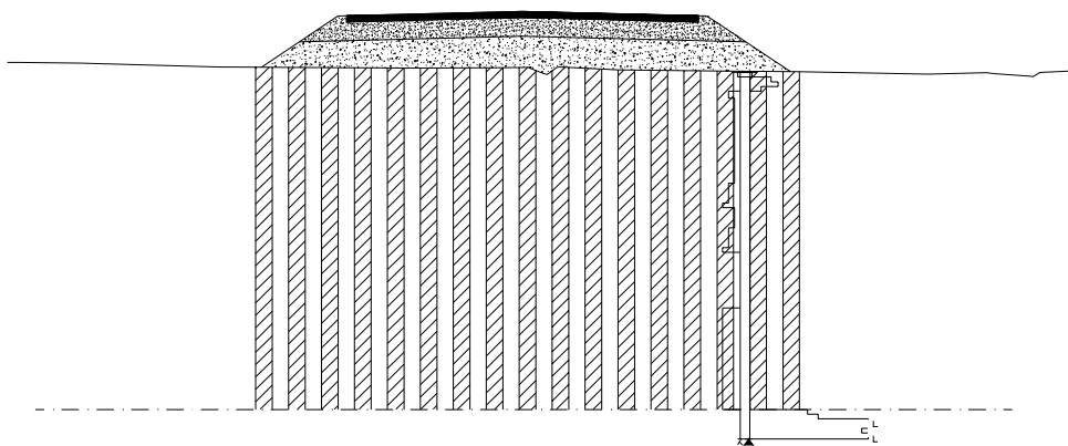
Kuva 6 Syvästabilointi pilareilla
