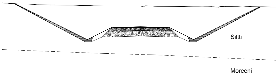
Kuva 8 Luiskaverhous silltileikkauksessa
