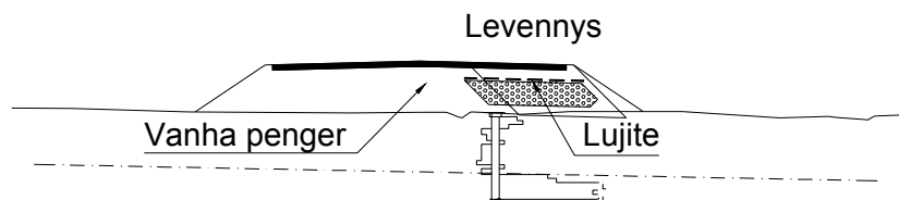
Kuva 4 Lujite pengerkevennyksen yhteydessä.
