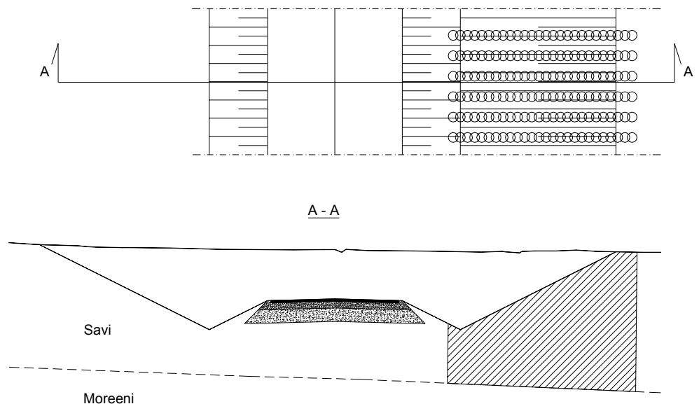
Kuva 11 Syvästabilointi luiskanvahvistuksena
