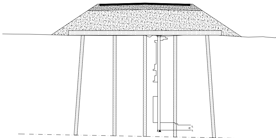
Kuva 7 Paalulaattarakenne
