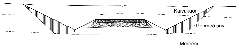
Kuva 9 Massanvaihto luiskassa
