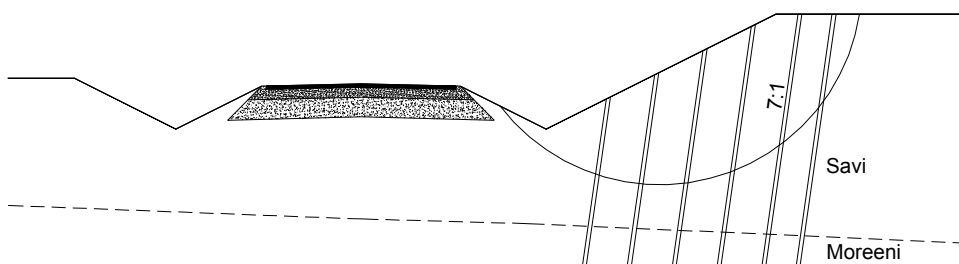
Kuva 12. Luiskapaalutus.
