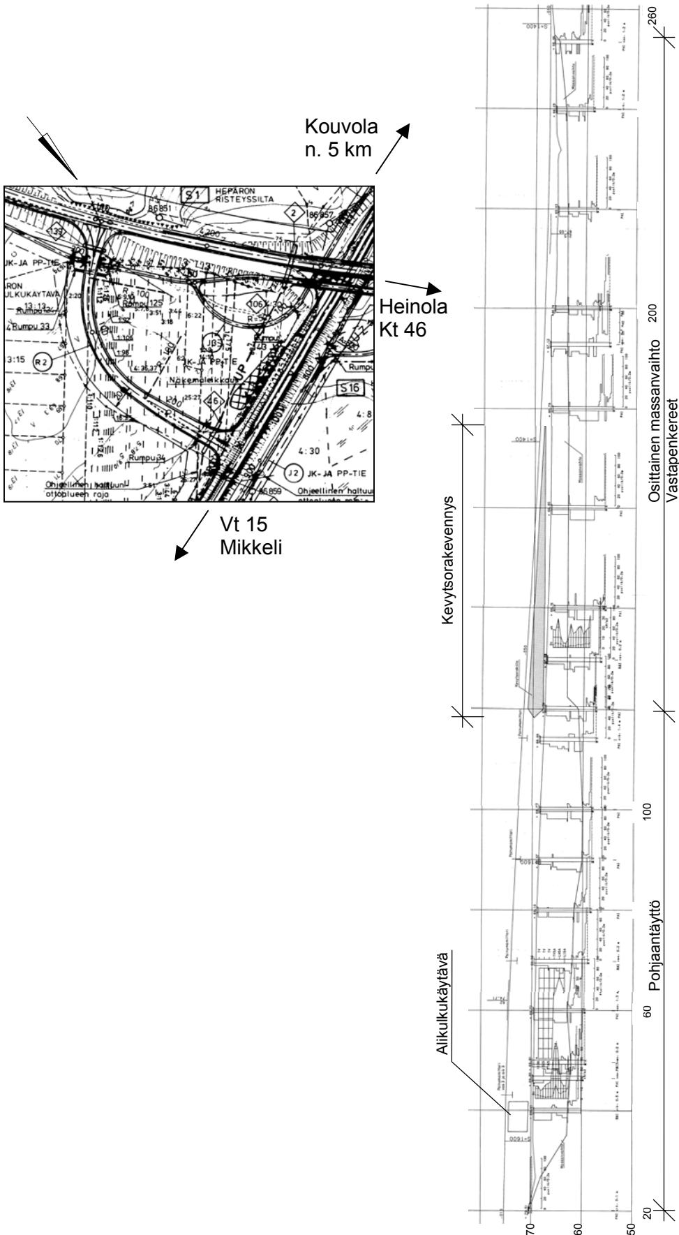
Kuva Kantatie 60 (nykyinen 46) välillä Heparo-Voikkaa, rampin E1/R2 kartta ja pituusleikkaus.
