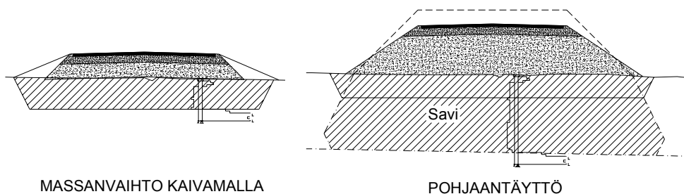
Kuva 5 Massanvaihto
