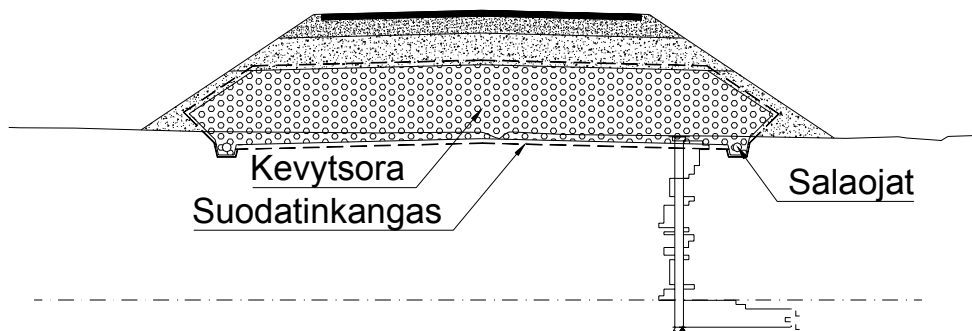
Kuva 3 Pengerkevennys
