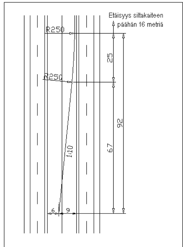
Kuva 19: Kaide keskialueella alikulkusillan kohdalla. Kaide käännetään keskialueelle viistoudessa 1:10.
