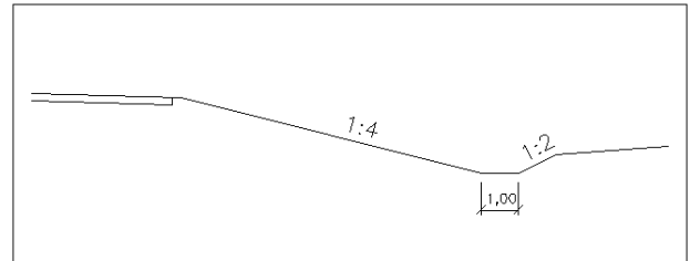
Kuva 1: Kaiteeton pengeri, vaihtoehtoisesti voidaan tehdä jyrkkä oja 2 – 6 metrin etäisyydelle luiskan alareunasta (etäisyys riippuu tien nopeudesta ja liikennemäärästä, kohdan 3 mukaisesti).
