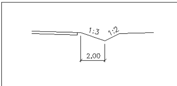
Kuva 9: Jyrkkä ojamuotoilu vähäliikenteisillä ja/tai alhaisen nopeustason teillä
