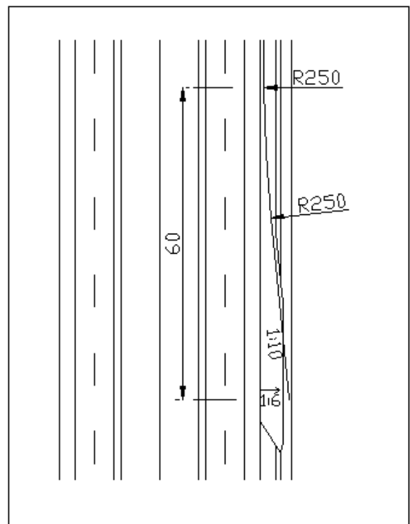
Kuva 20: Kaiteen pään kääntäminen ulkoluiskaan
