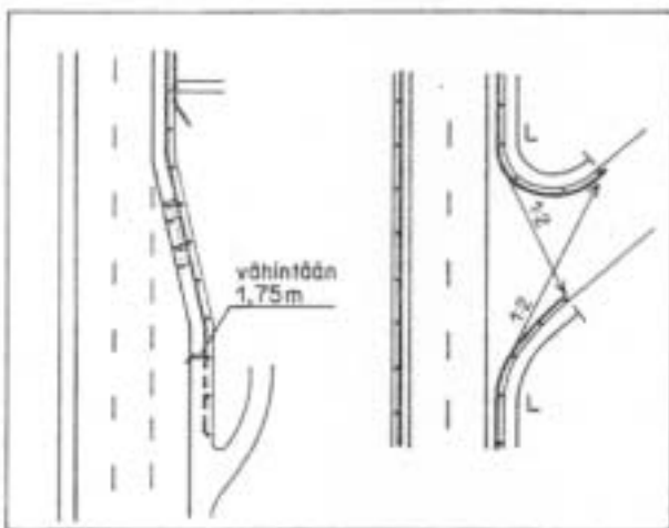
Kuva 21: Kaiteen aloittaminen pysäkin kohdalla ja kaidteen päiden kääntäminen vähäliikenteiselle sivutielle.
