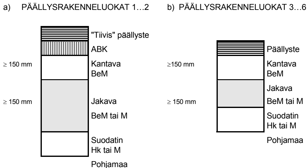
Kuva 2.1: Tyypillinen betonimurskerakenne (BeM=betonimurske). a) Päällysrakenneluokkien 1...2 ja b) päällysrakenneluokkien 3...6 betonimurskerakenne. "Tiivistä" päällystettä suositellaan käytettäväksi kohdan 7.6 periaatteiden mukaisesti korkealuokkaisilla teillä.
